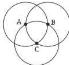
A, B ଓ C ସମବ୍ୟାସାର୍ଦ୍ଧ ବିଶିଷ୍ଟ ତିନୋଟି ଦୃଢ଼ର କେନ୍ଦ୍ରବିନ୍ଦୁ ।
