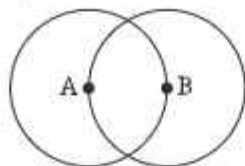
A ଓ B ଦୁଇଟି ସମବ୍ୟାସାର୍ଦ୍ଧ ବିଶିଷ୍ଟ ଦୃଢ଼ର କେନ୍ଦ୍ରବିନ୍ଦୁ ।
