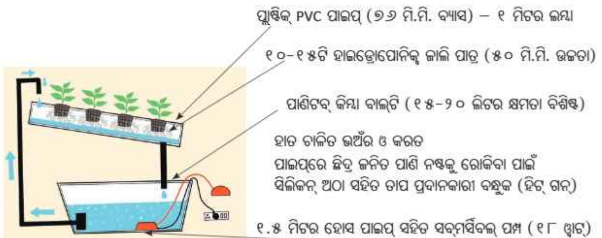
ଚିତ୍ର ୧.୩ (ଗ) : (NFT) ହାଇଡ୍ରୋପୋନିକ୍ସ ବ୍ୟବସ୍ଥା
